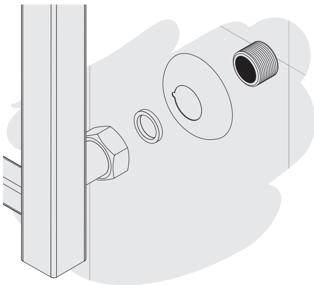
Вариант подключения через накидные гайки
