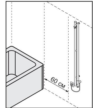
Полотенцесушитель установлен на расстоянии >60 см от края ванны или душевой кабины.
