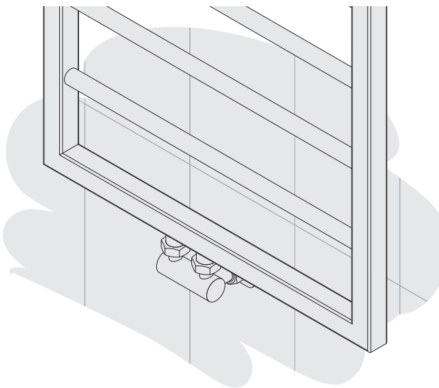
Вариант нижнего подключения EU50 через модуль
