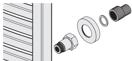
Вариант нижнего подключения через носики
