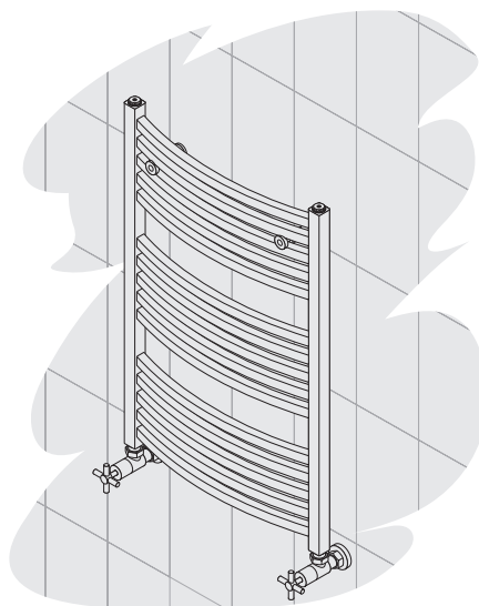
Вариант нижнего подключения через вентили
