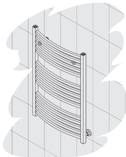
Вариант нижнего подключения через носики
